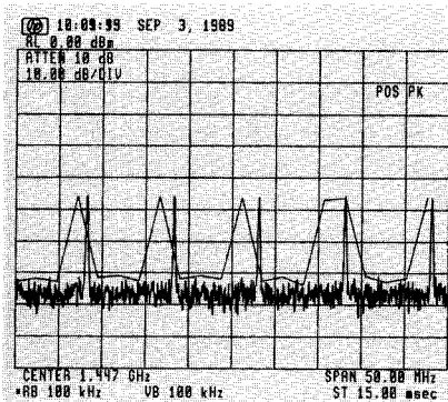
Fig. 35. Pos peak display mode versus actual comb.
